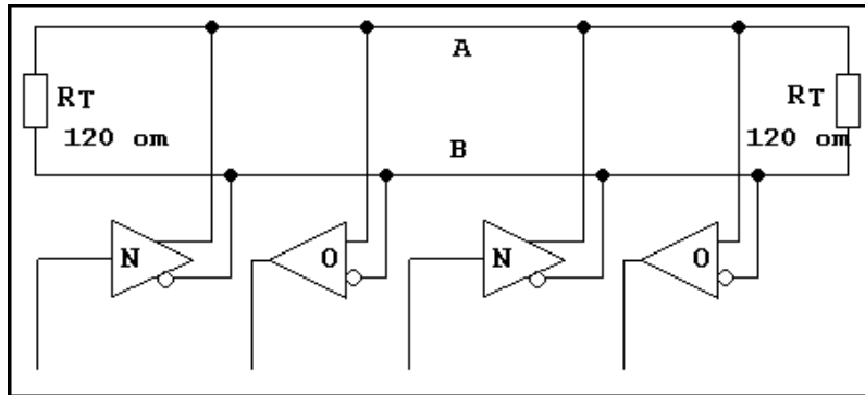
Rys.1 Rezystory dopasowujące RT
